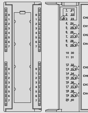
6ES7 331-7NF00-0AB0
