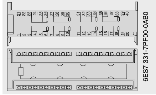
Bild 2/5 Analogeingabebau- gruppe SM 331-7PF00
