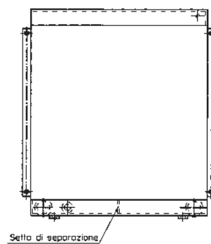
Setto di separazione Flow separator P/N 2G7012### P/N 2G7024###
