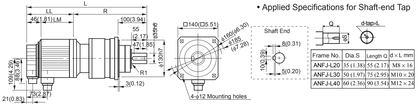
ANFJ-L30
