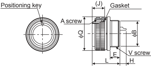
(d) Plug
