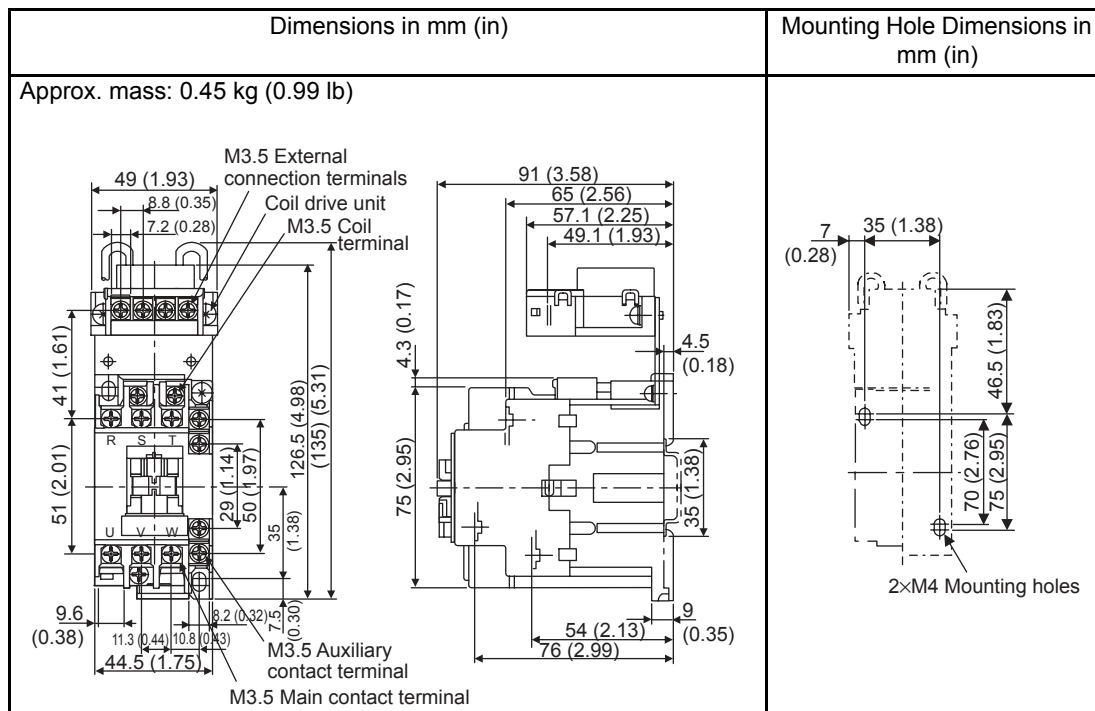
(d) Model: HI-25JCU and HI-35JCU
