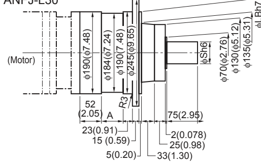
ANFJ-L30
