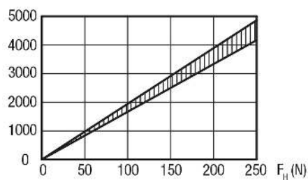
Silový diagram
