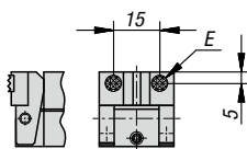
2 insertos de metal duro cuadrados y prisma
