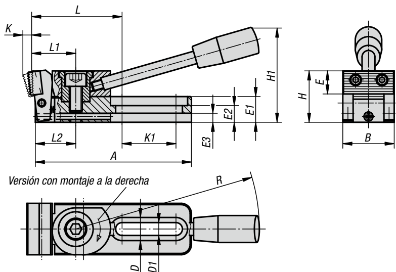
Forma A Mordaza de sujeción de acero acanalada
