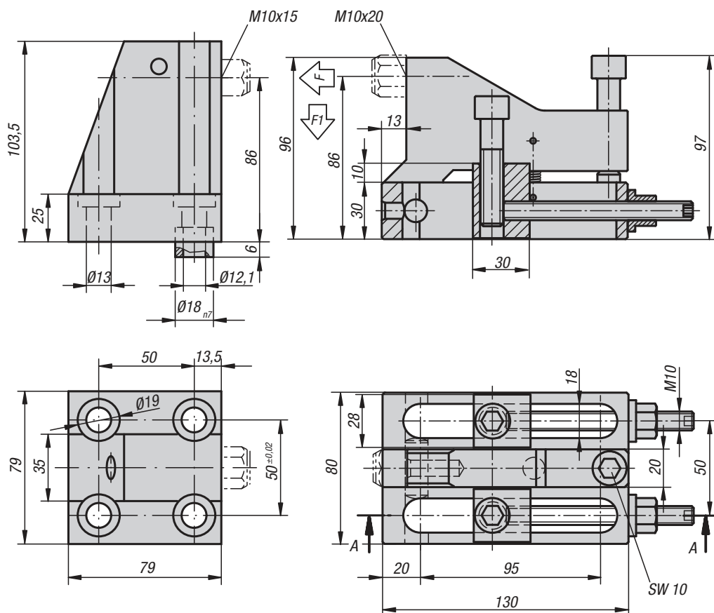
K0830.112 A-A
