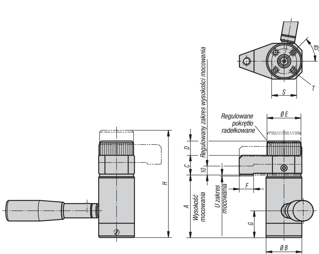
Wykonanie prawostronne
