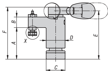
Wykonanie prawostronne
