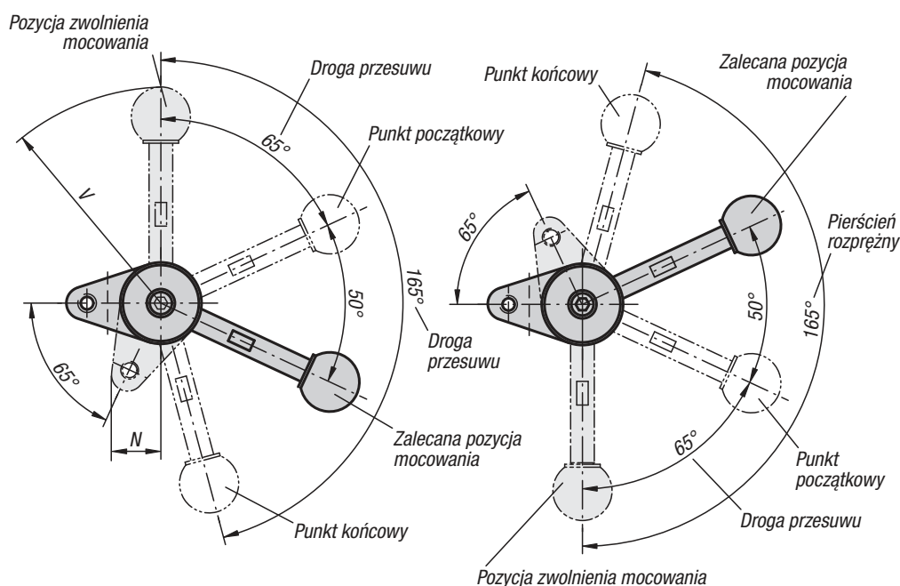
Wykonanie prawostronne
