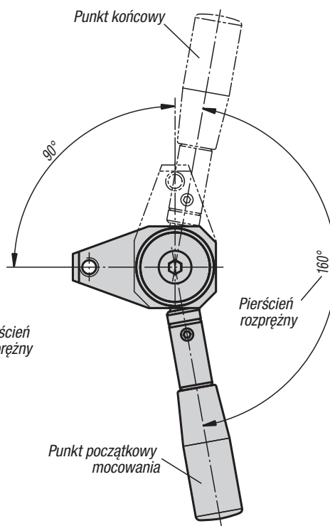
Wykonanie lewostronne
