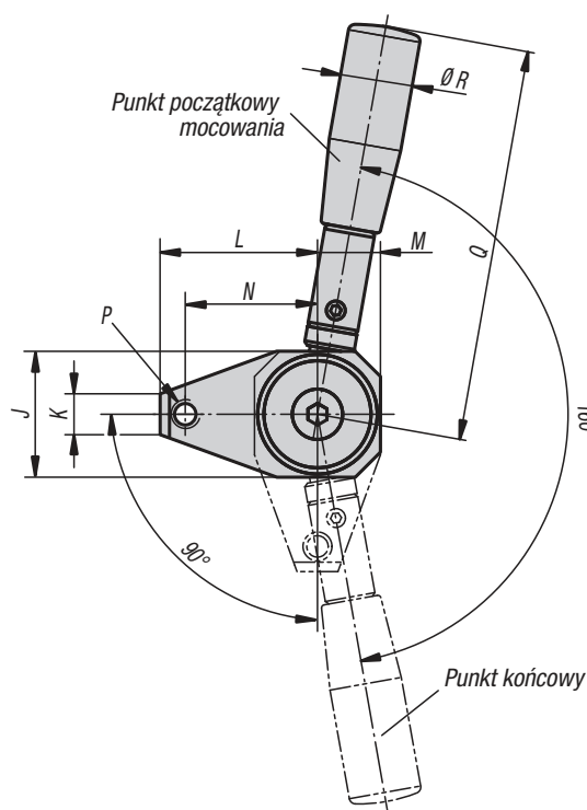
Wykonanie prawostronne
