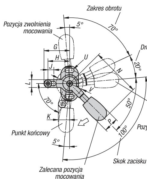
Wykonanie prawostronne
