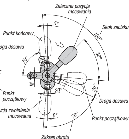
Wykonanie lewostronne
