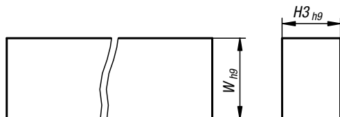
Установочные размеры для ответной детали квадратной головки
