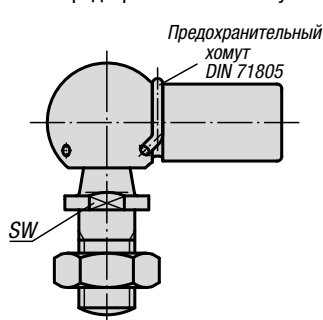
Форма CS с предохранительным хомутом
