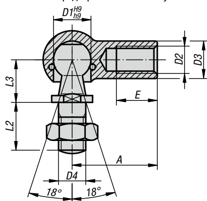
Форма С без предохранительного хомута
