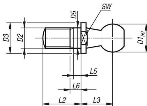
Форма С с резьбовой цапгой SW
