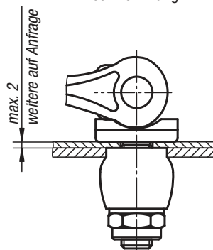
Blechklemmung 2
