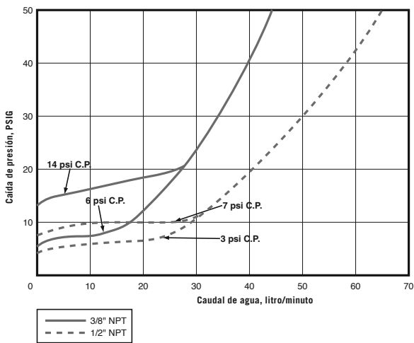
Modelos con conexiones hembra NPT 3/8" y 1/2"
