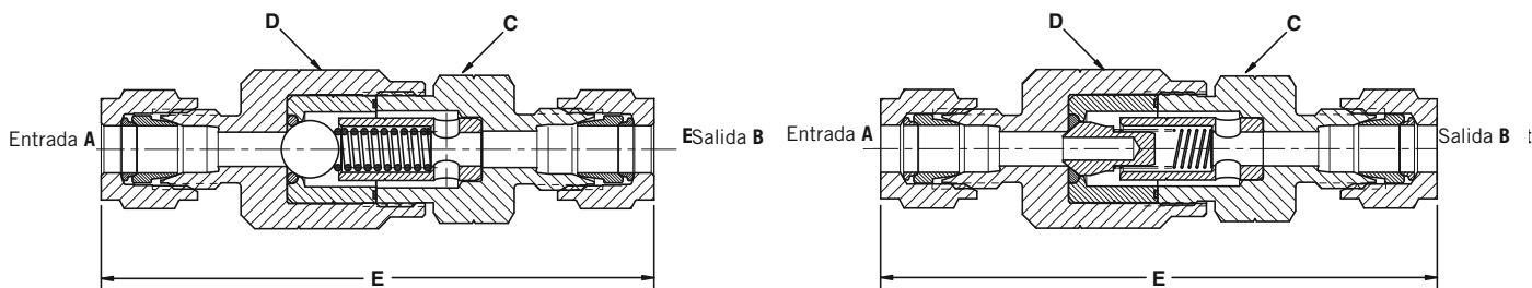
Válvulas de retención de bola serie 6100
