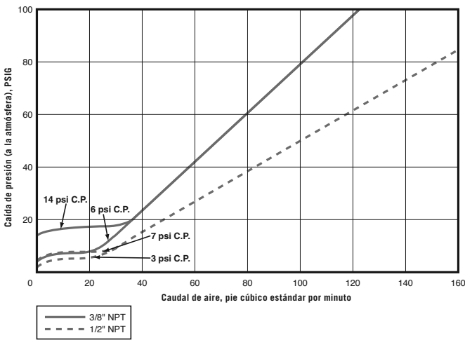
Modelos con conexiones hembra NPT 3/8" y 1/2"
