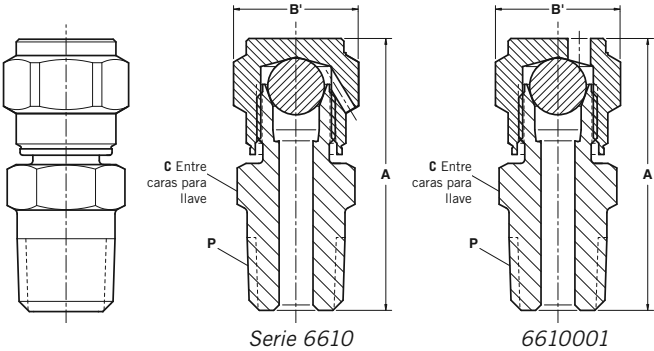
Serie 6610: válvulas rectas (montadas sobre salida directa)
