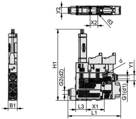
Tasarım verileri SCPSb 2-09 S04 NO VD
