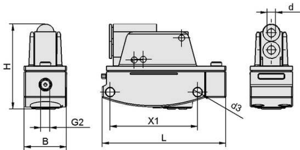
Konstruktionsdaten VS-V-PM-NC
